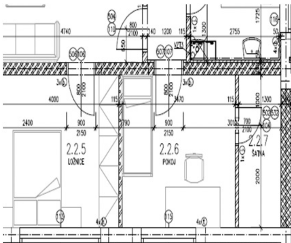
Obr. Výřez jedné bytové jednotky
